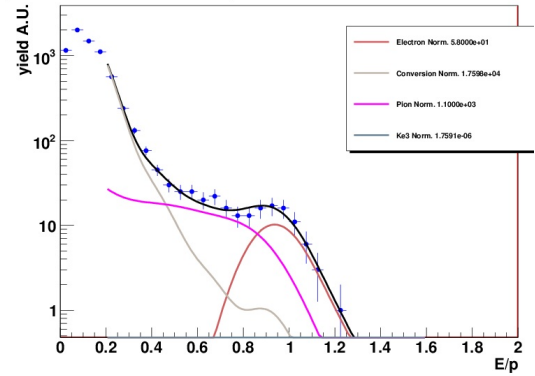
E/p (10.0-11.0)GeV p_T bin
